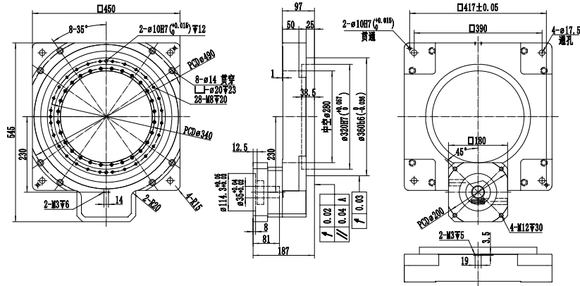
Dimension(motor shaft OD 35mm)
