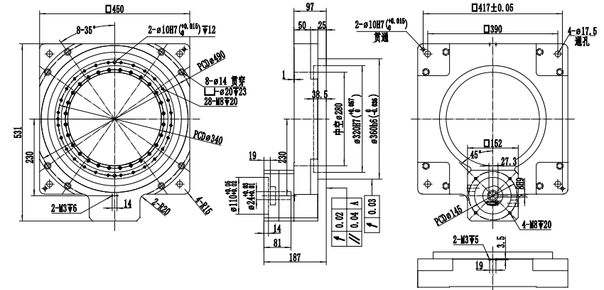
Dimension(motor shaft OD 24mm)
